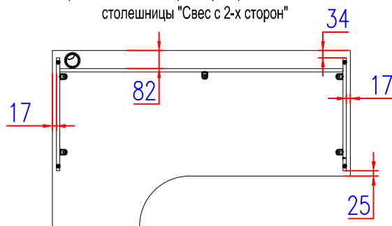
Вид сверху (Исполнение 1) рекомендованные размеры при положении столешницы "Свес с 2-х сторон"
