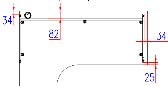
Вид сверху (Исполнение 1) рекомендованные размеры при положении столешницы "Свес слева"
